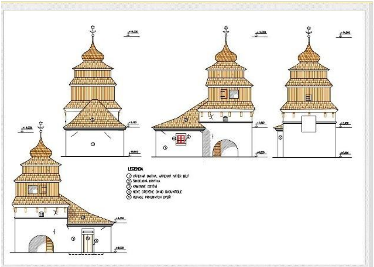
Semanín, projekt rekonstrukce barokní márnice při zvonici – výkresová dokumentace
